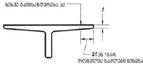
სურათი 721.2.2.1.2 ფილის სისქის განსაზღვრა დამრეცი სოფიტებისთვის
