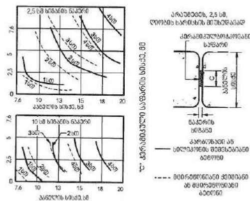
სურ. 722.2.1.3.1 კერამიკ-ბოჭკოს ბმულის დამცავი
