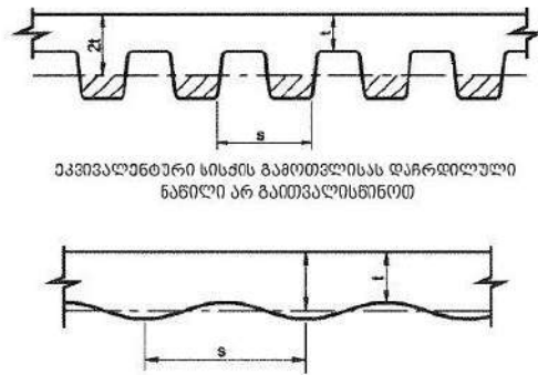
სურათი 722.2.2.1.3 ფილები დაღარული ან ტალღოვანი სოფიტებით
