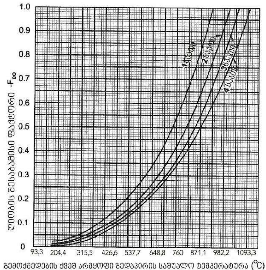
სურათი 705.7 ღიობის ეკვივალენტური ფაქტორი
